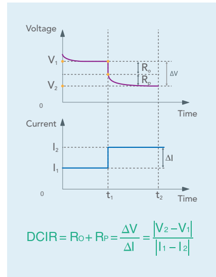
DCIR Test (2)
