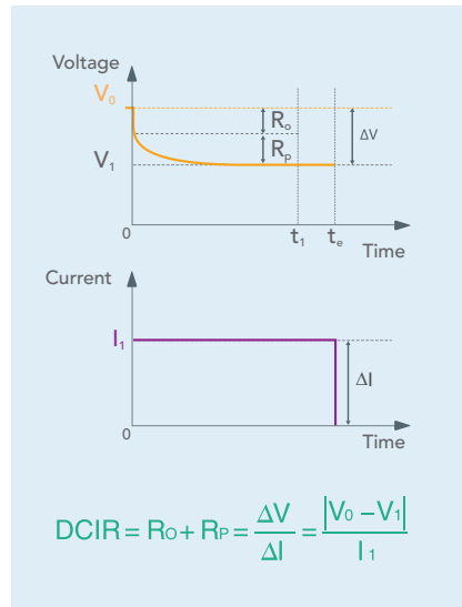
DCIR Test (1)
