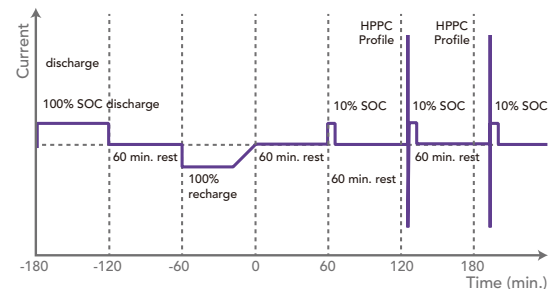
HPPC Test
