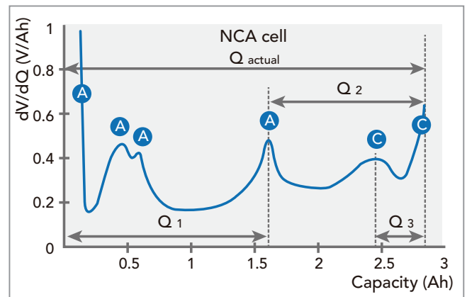
dV/dQ Test
